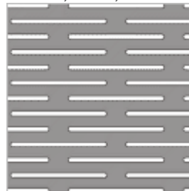
отверстие 1 x 20мм Шаг 3,2 x 2,4мм
