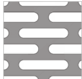
отверстие 5 x 25мм Шаг 8 x 30мм
